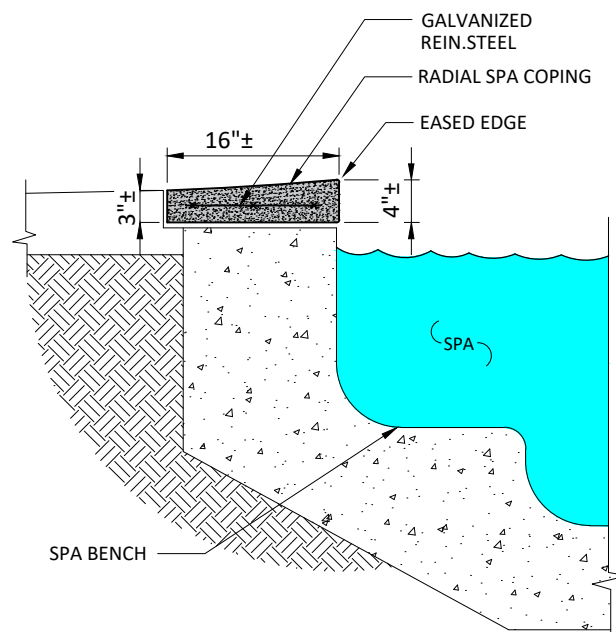
Typ. Spa Section
