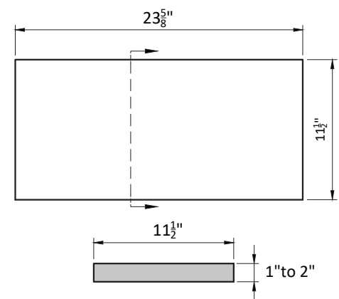
SQUARE EDGE COPING
