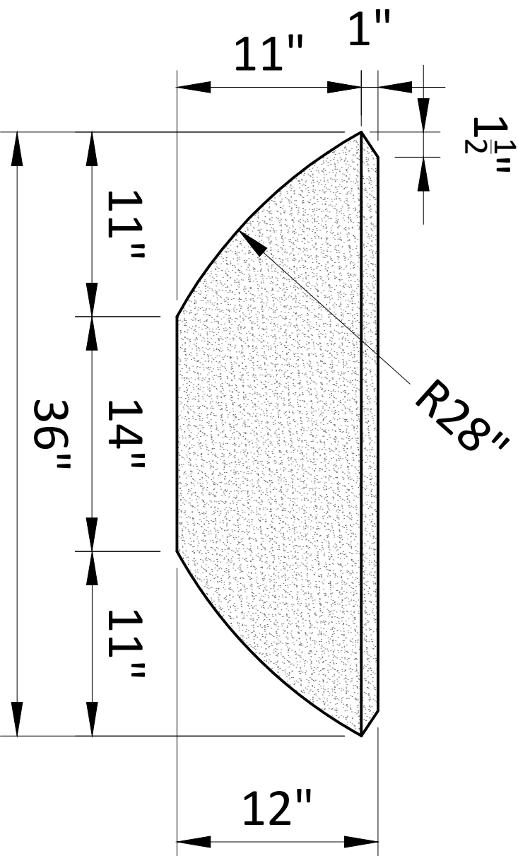
36"Dia.x 12" Ht.Planter
