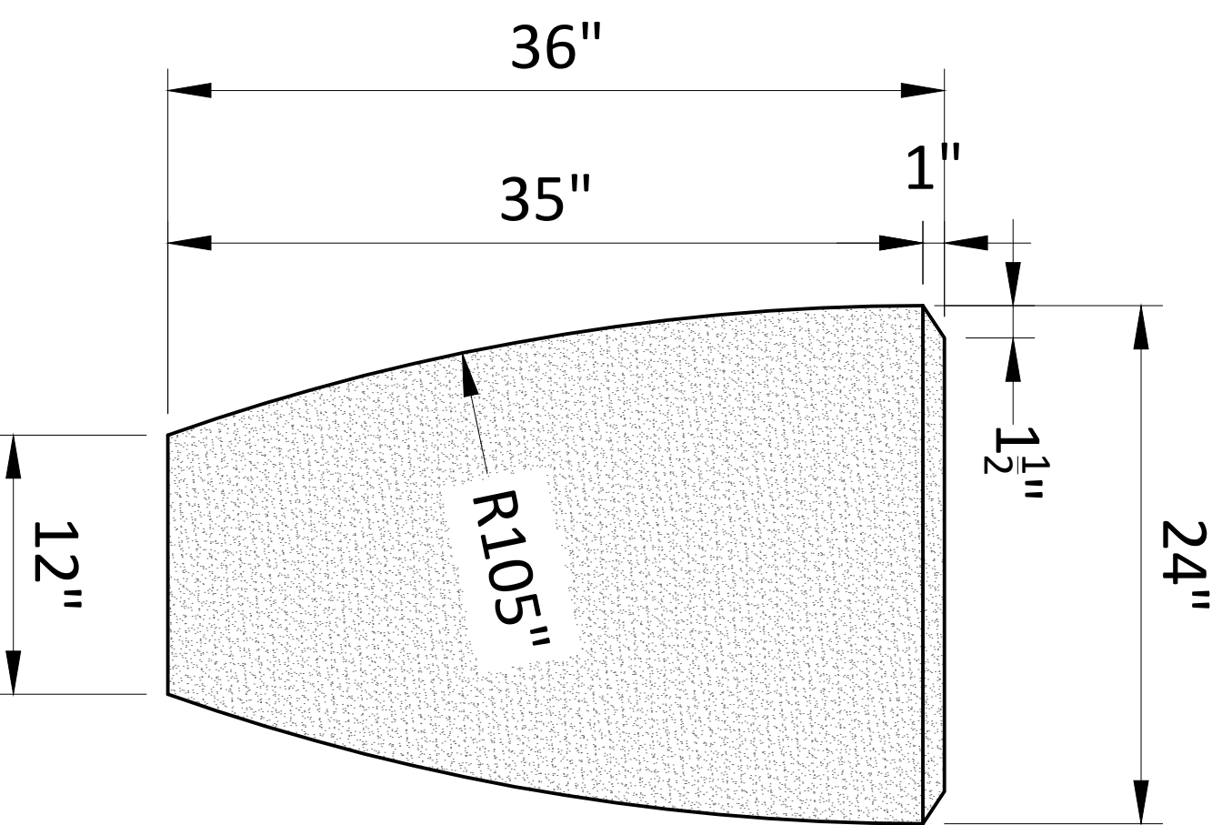
24"Dia.x 36" Ht.Planter
