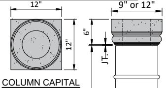
COLUMN CAPITAL
