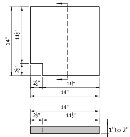
SQ. EDGE COPING CORNER
