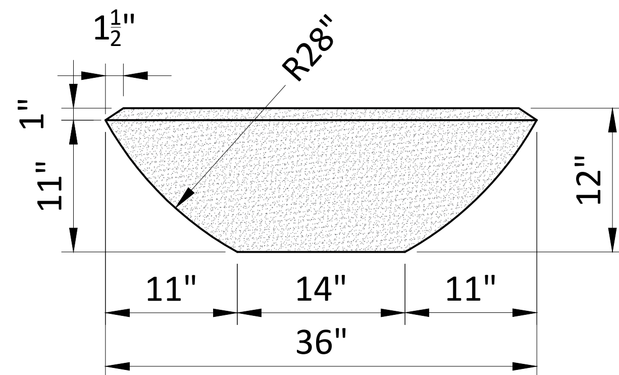
36"Dia.x 12" Ht.Planter
