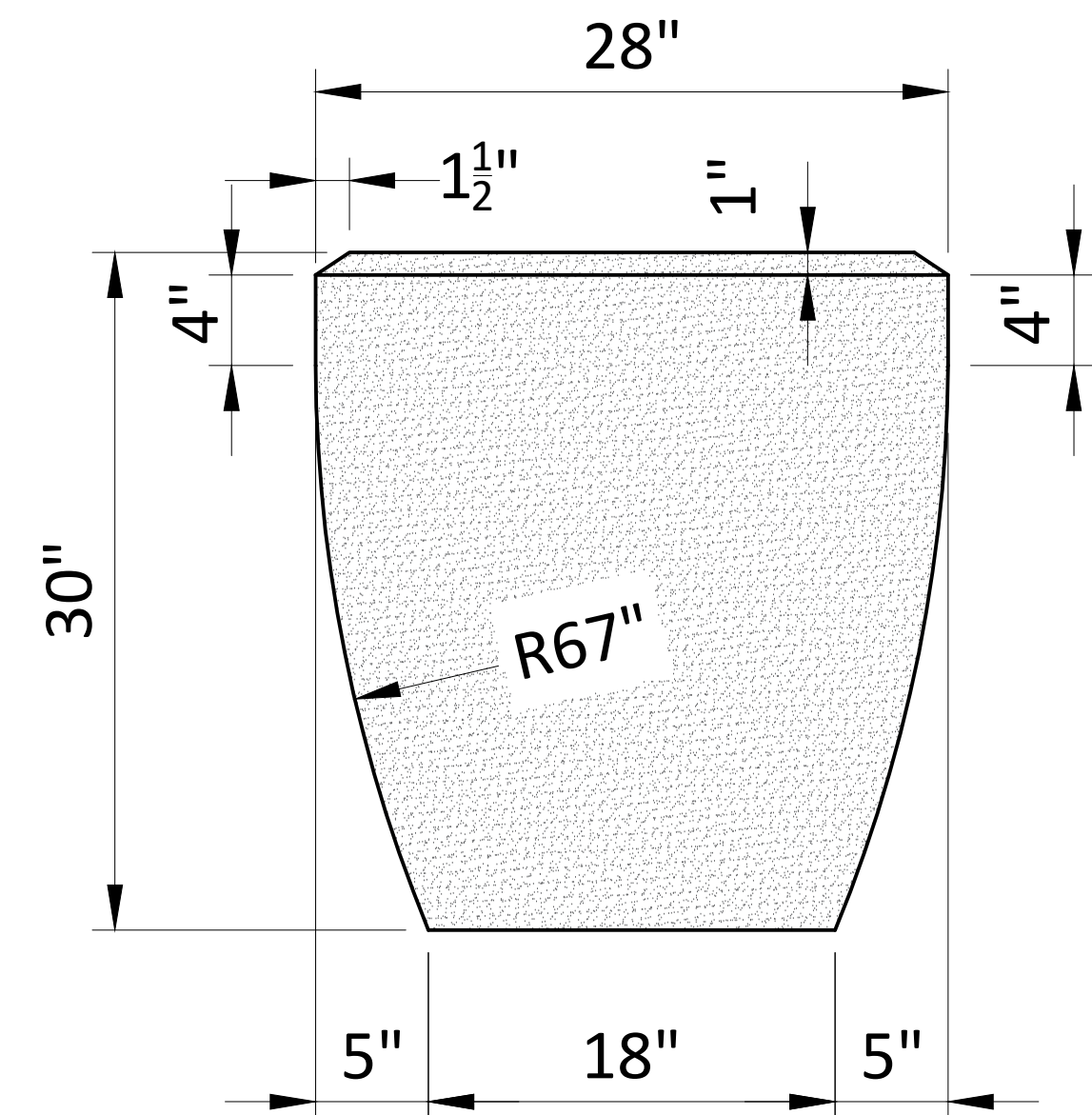
28"Dia.x 30" Ht.Planter
