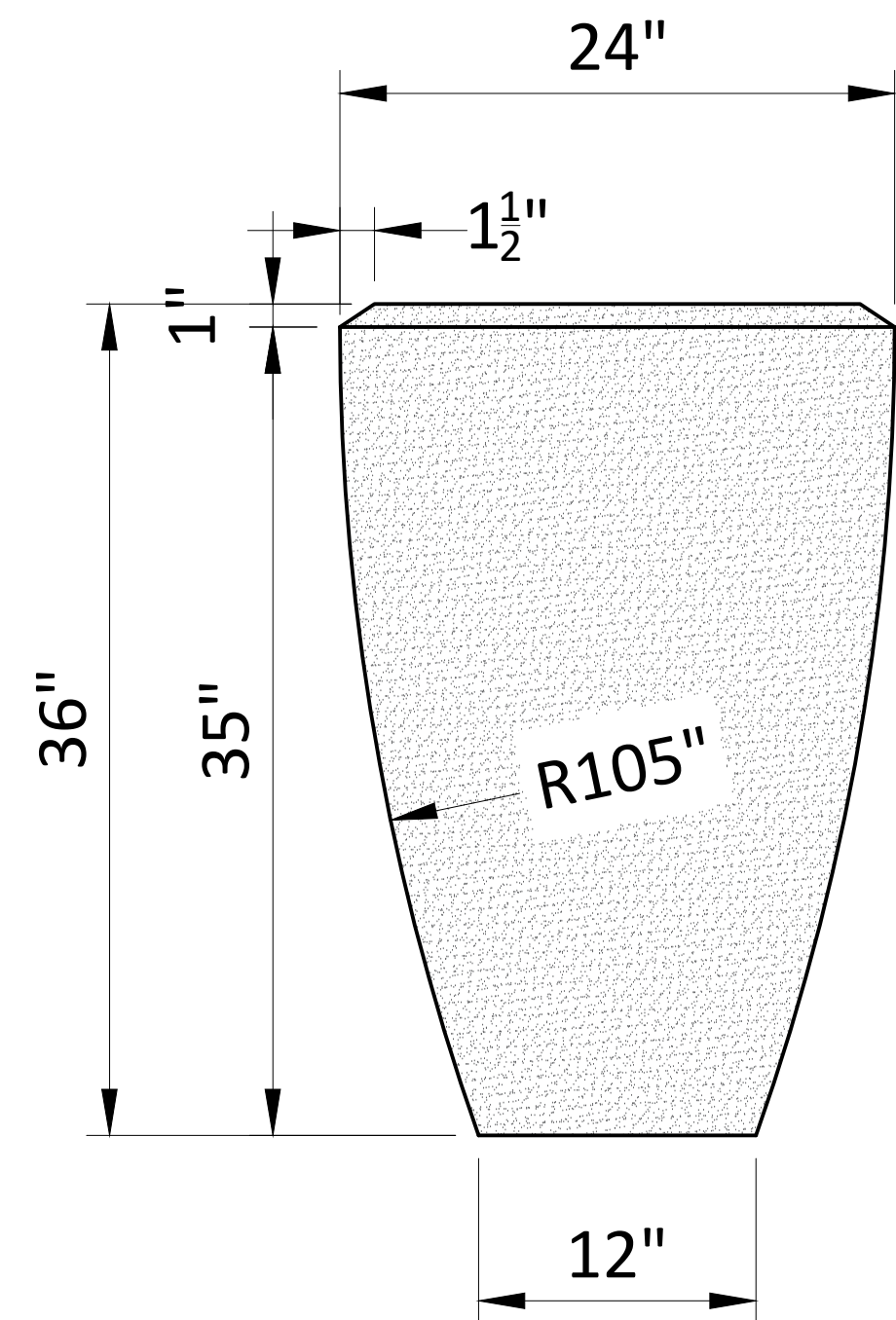
24"Dia.x 36" Ht.Planter
