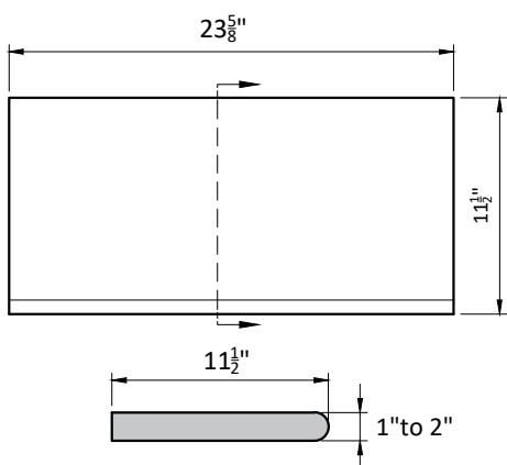
Typ. Skimmer Pad
